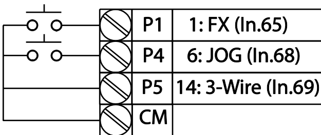
[Klemmenanschlüsse bei 3-Leiter-Betrieb]
